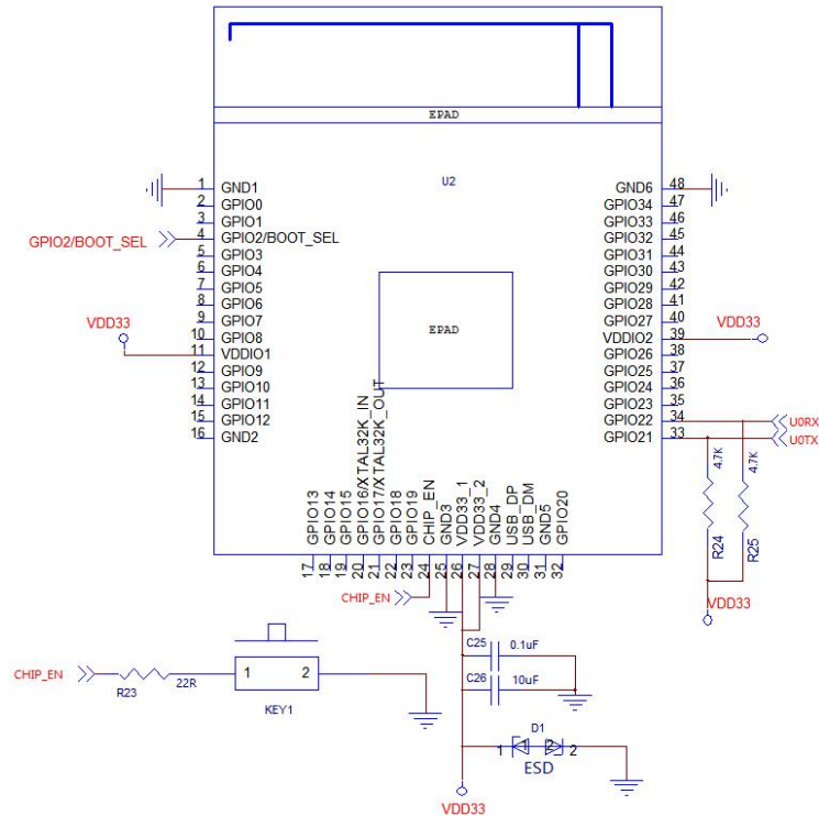
图 11 应用指导电路
