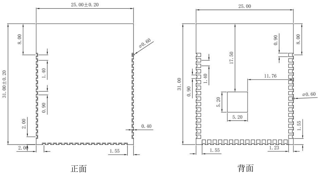
图 4 尺寸图
