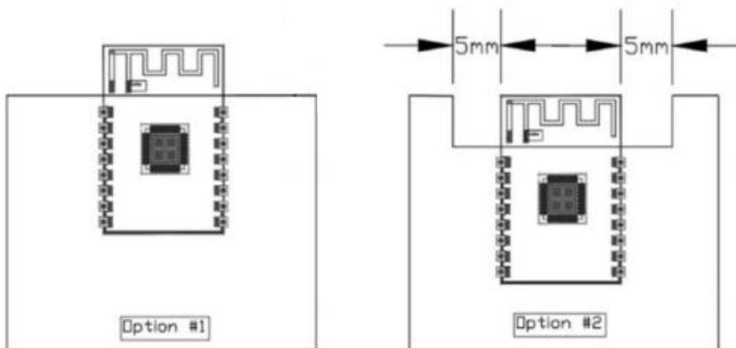
图 13 天线布局示意图
