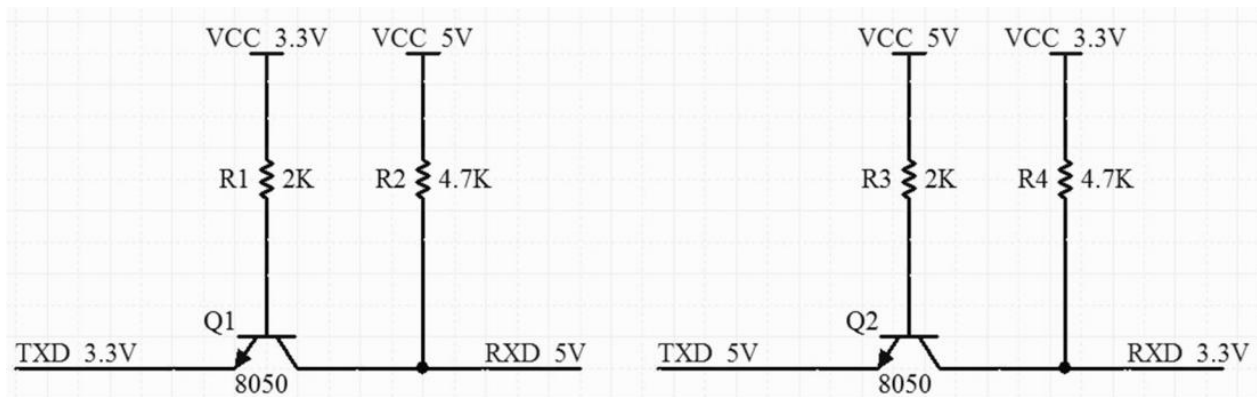
图 15 电平转换电路
