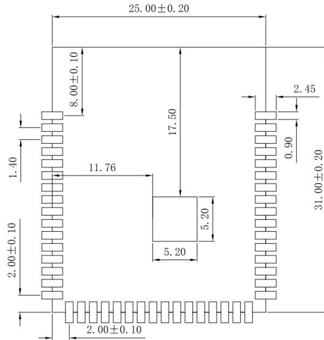
图 12 推荐 PCB 封装尺寸
