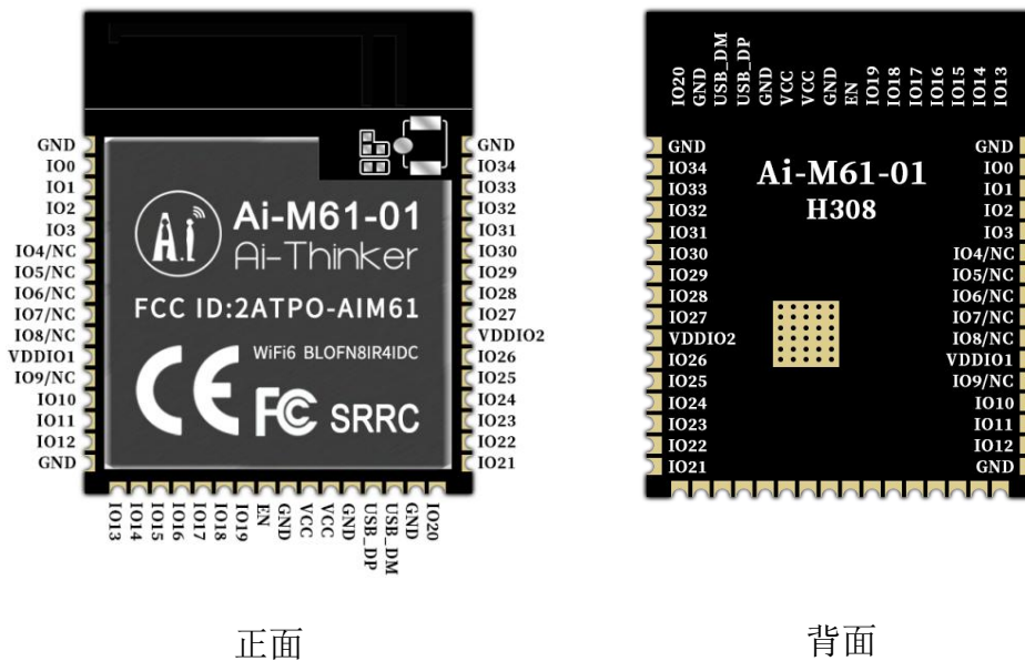
图 6 管脚示意图
